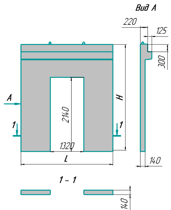
Рисунок с одной полкой и проемом
