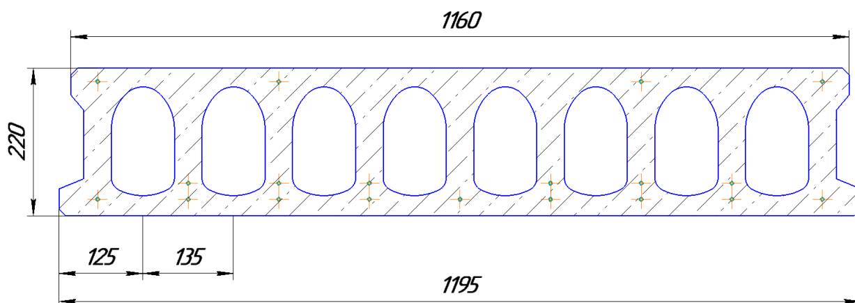
Номенклатура пустотных плит по альбому ИЖ 568-03 высотой 220мм.
