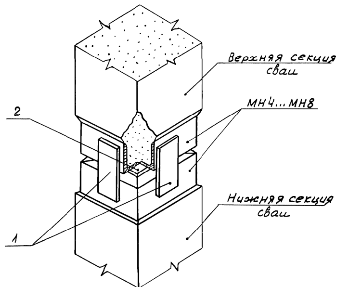
Рис 2. Стаканный стык составной сваи.
