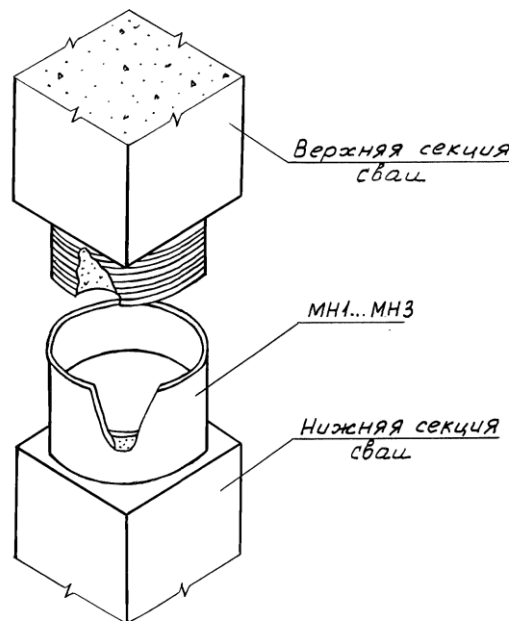
Рис 2. Стаканный стык составной сваи.
