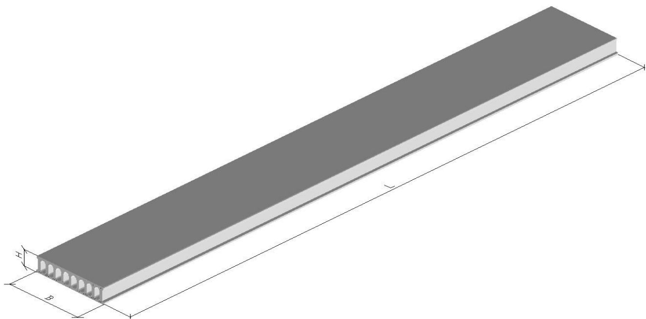
Плита ПБ
