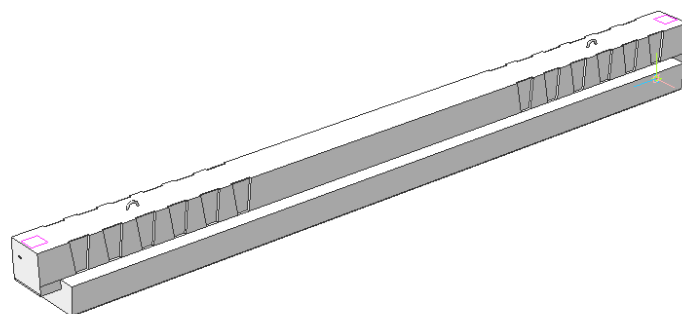
Рис. 2. Сечение ригелей РДП 4.26; 56; 68. и РДП 4.27; 57; 69.
