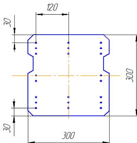
Сечение свай
