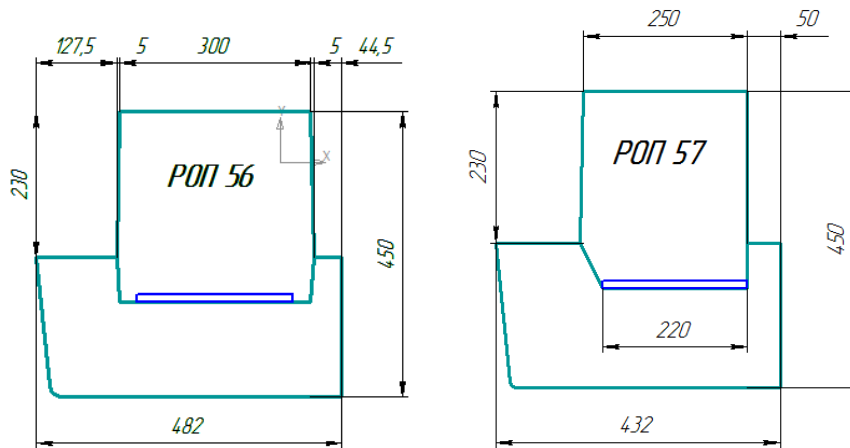
Рис. 4. Сечение ригелей РОП 4.26; 56; 68.и РОП 4.27; 57; 69.
