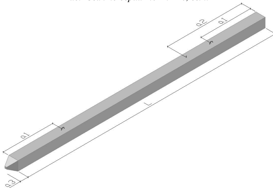
Рис. Свая по серии 1.011.1-10, вып.1
